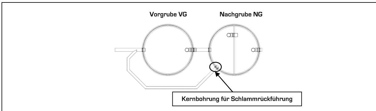
Bsp.1: Schlammrückführung Alternative 1 (Verlegt bis in den Zulauf des ersten Behälters)
